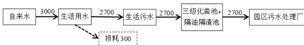
图 1 项目水平衡图（单位：m 3 /a）
