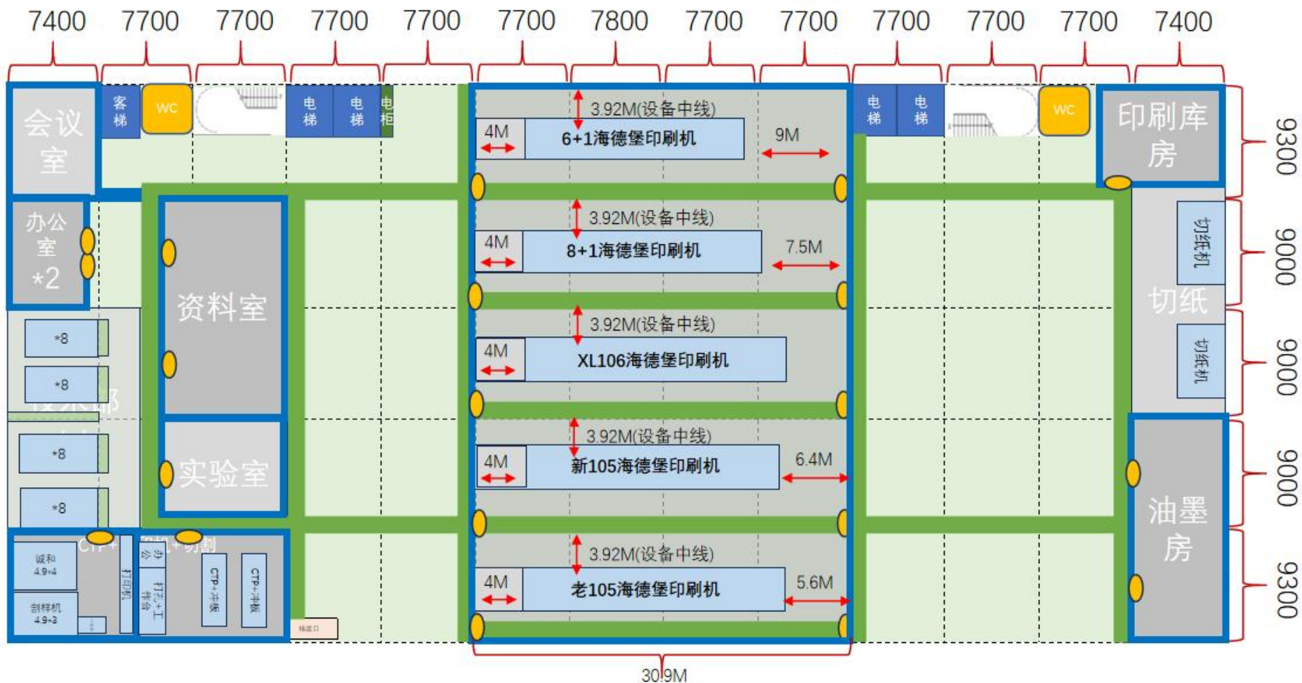
附图 4-2 项目 1# 厂房 2F 车间平面布置图
