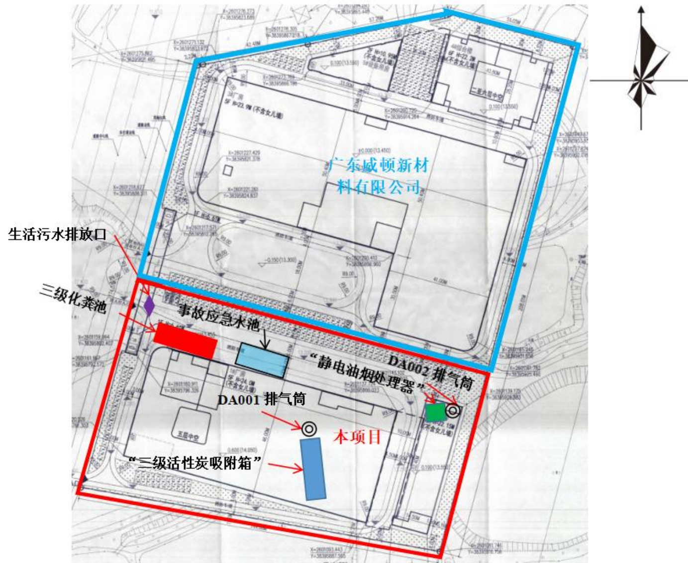
附图 5 项目总平面布置图
