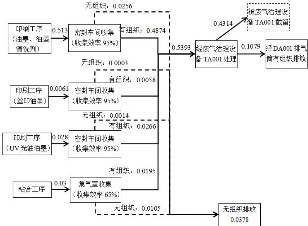
图 2 项目 VOCs 平衡图 (单位: t/a)
