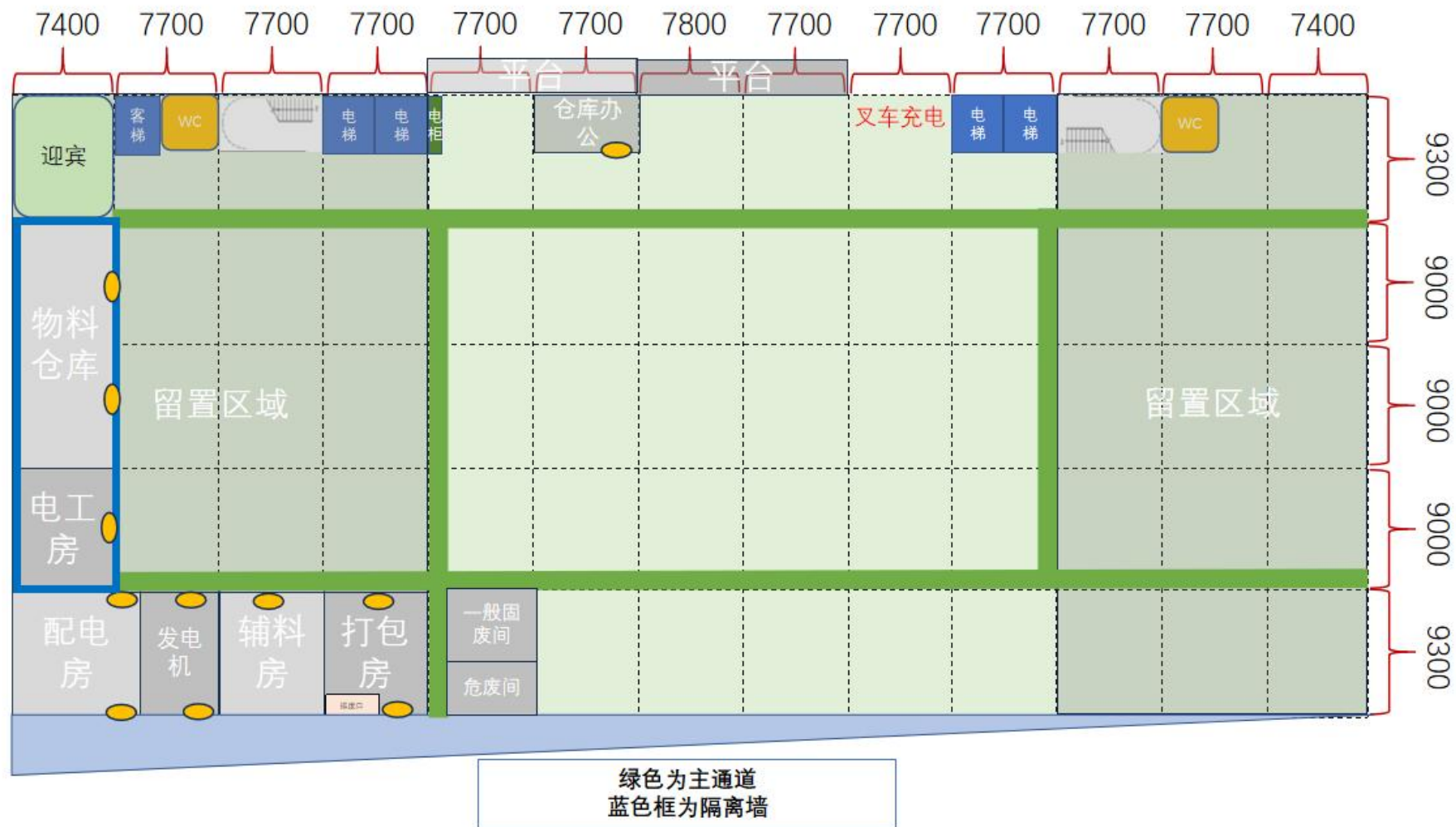
附图 4-1 项目 1#厂房 1F 车间平面布置图
