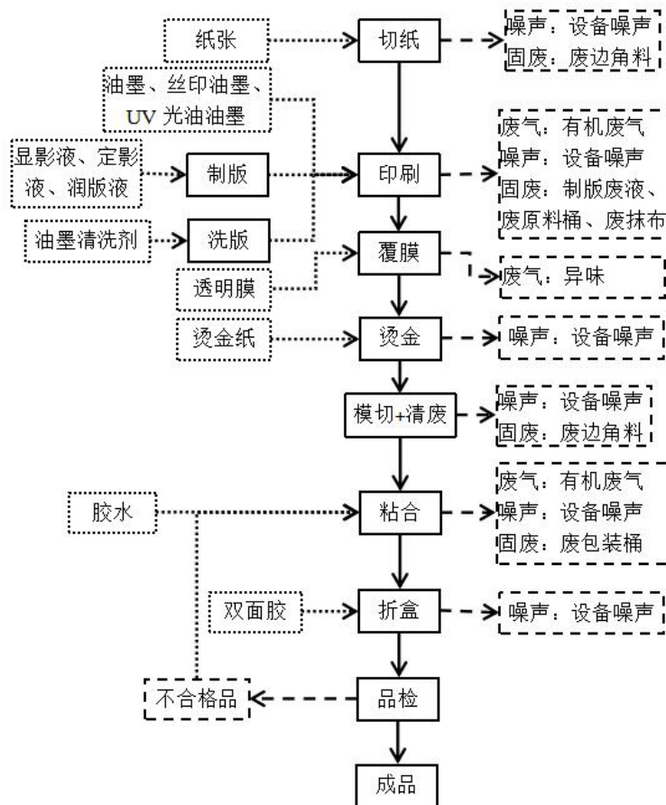
图 3 项目化妆品包装盒、药品包装盒、彩卡和说明书生产工艺流程图
